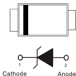
TSP5L60AF SMAF
